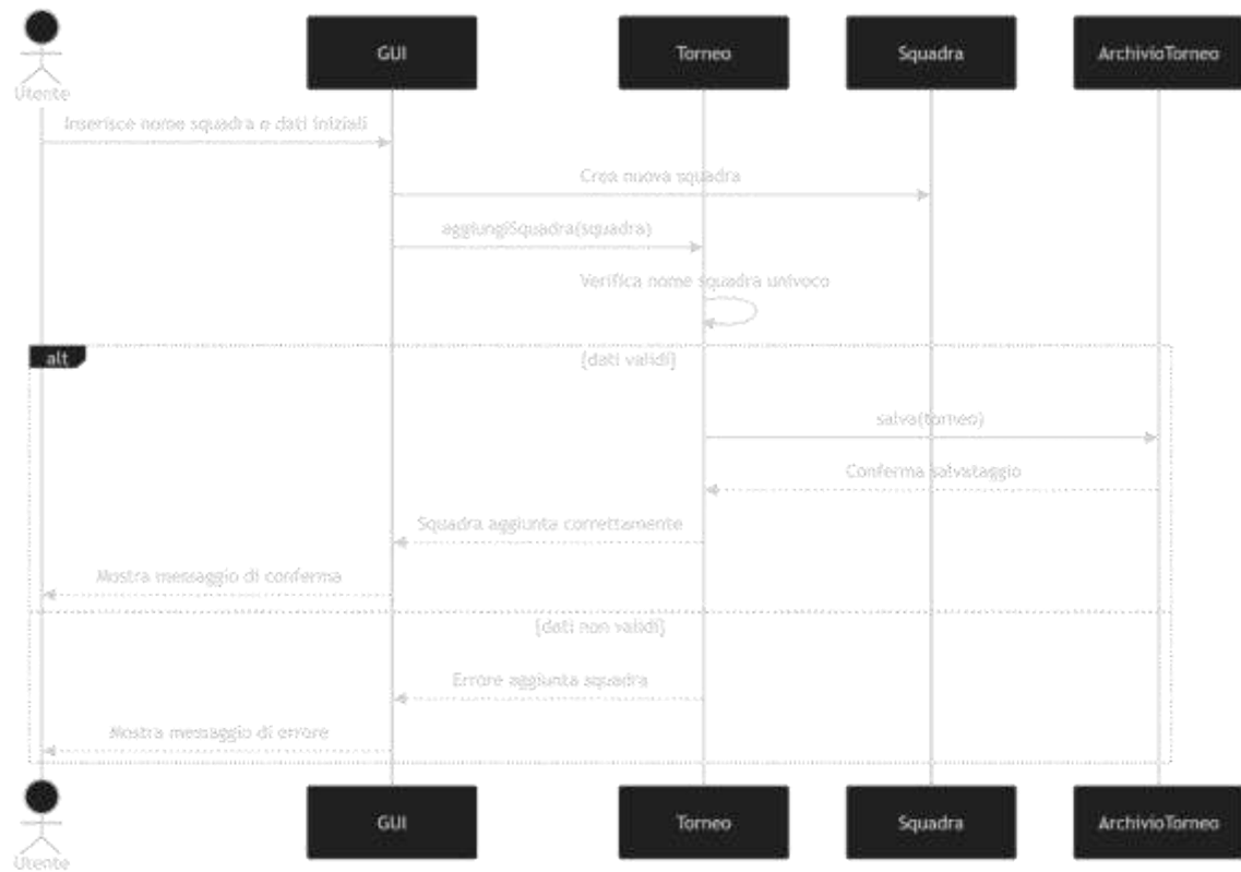
Diagramma di sequenza: aggiunta squadra
