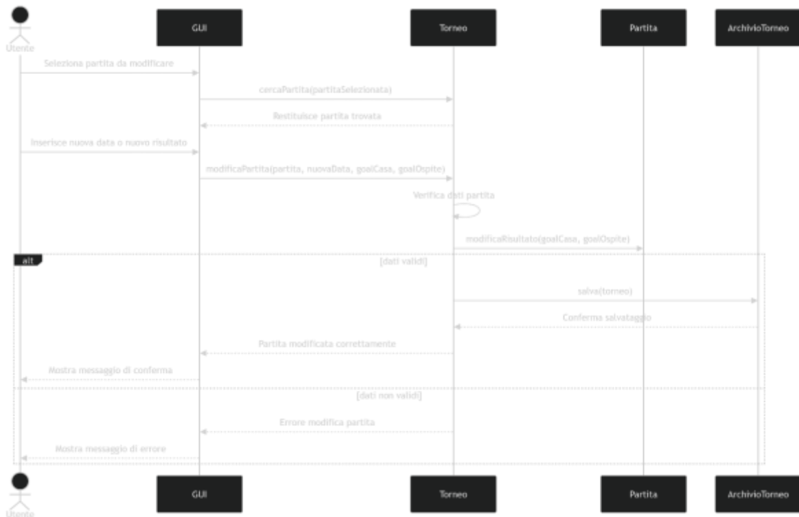
Diagramma di sequenza: modifica partita
